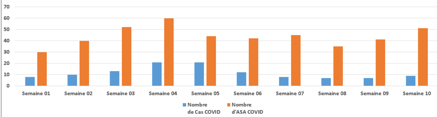
Evolution du nombre de cas COVID et cas ASA COVID par semaine - DEE Période du 01 janvier au 12 mars 2021
